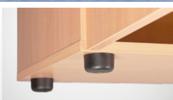
Rektifikálás – a mellékelt imbuszkulcs segítségével könnyen megoldható az egyenetlen padló
