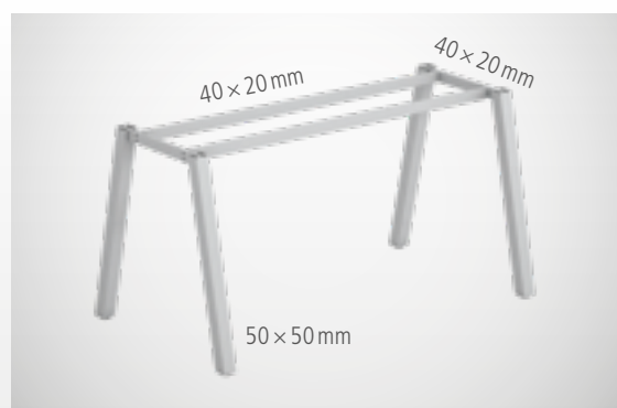
Lábzat UNI A (20. old.)
