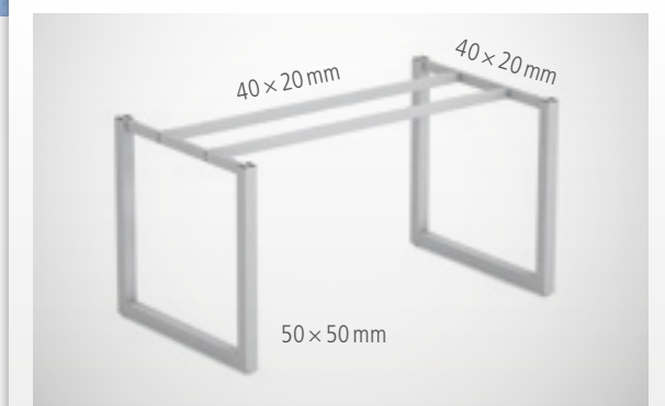
Lábzat UNI O (24. old.)
