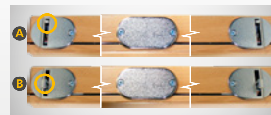
Kétpontos zár az ajtóba marott rudakkal
